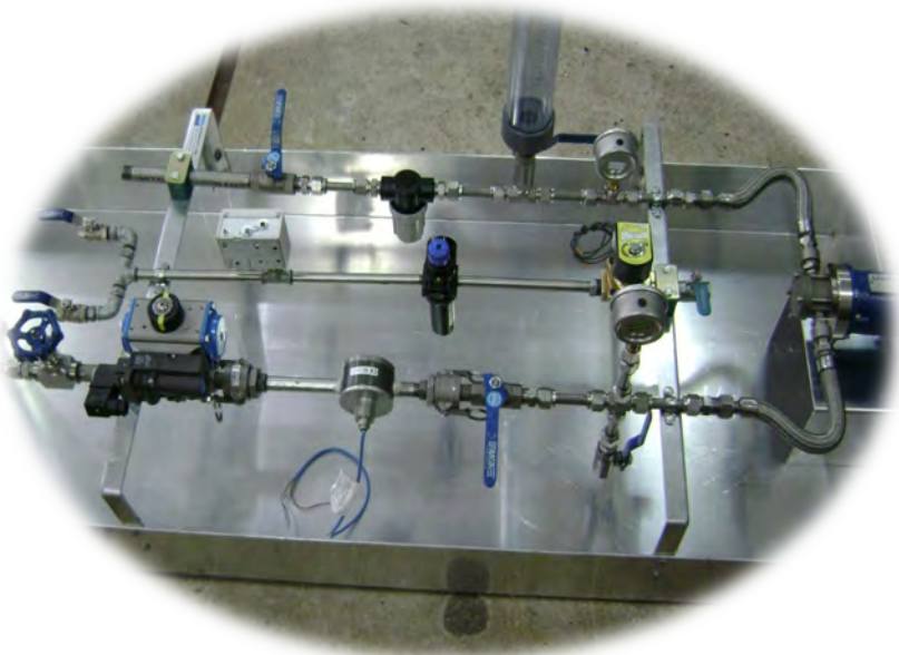
Injeção de Anti-Salmonela em Rações Animais - Sadia Btech
